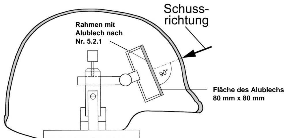
Seitenansicht
