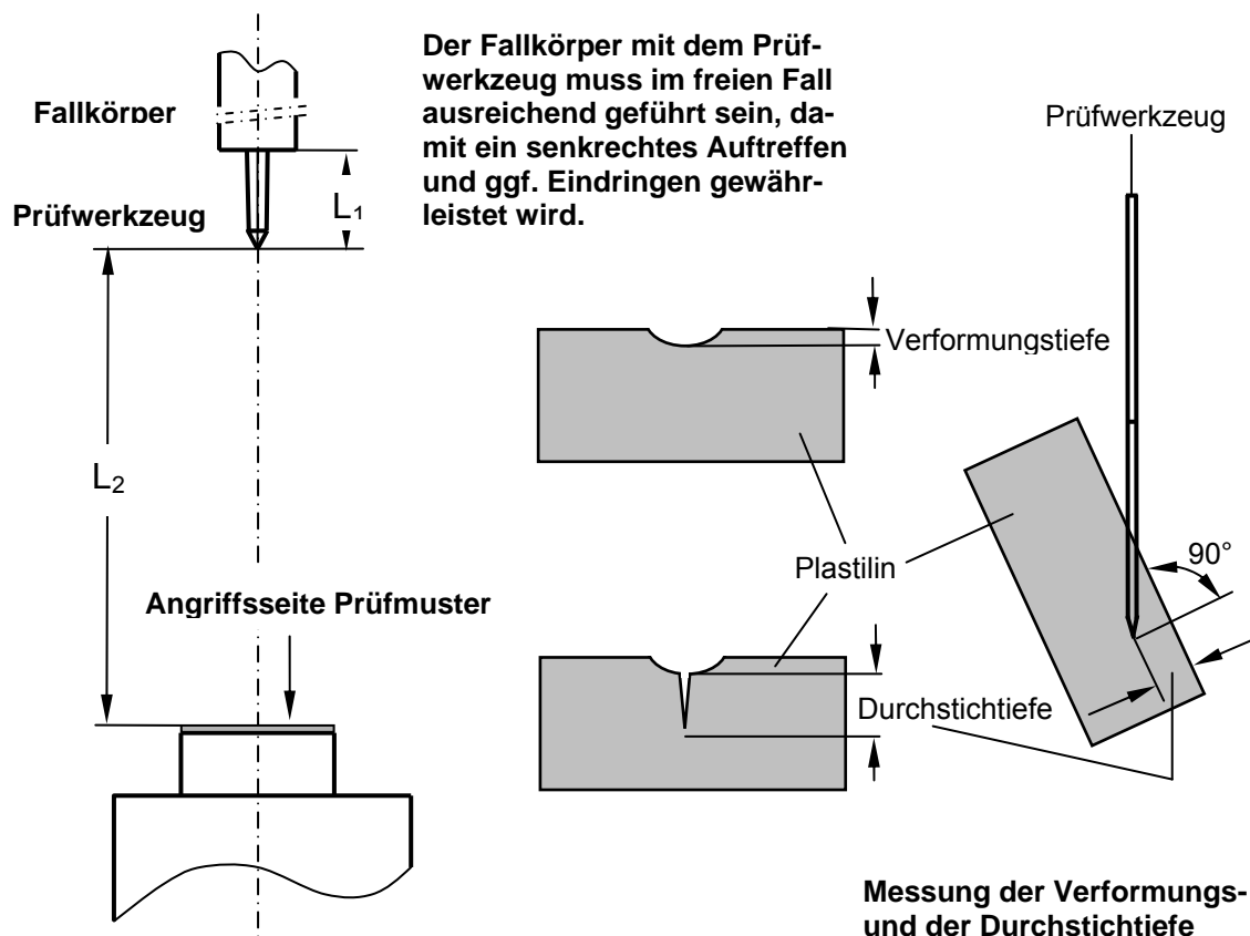
Zeichnung 4: Fallprüfgerät
