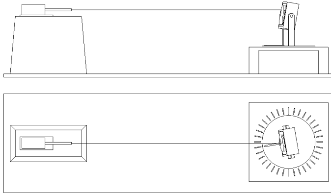
Abb. 1: Auftreffwinkel 80°/80° (Plastilinkasten 10° horizontal gedreht sowie 10° vertikal gekippt)
