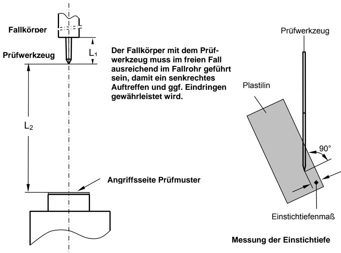
Zeichnung 4: Fallprüfgerät
