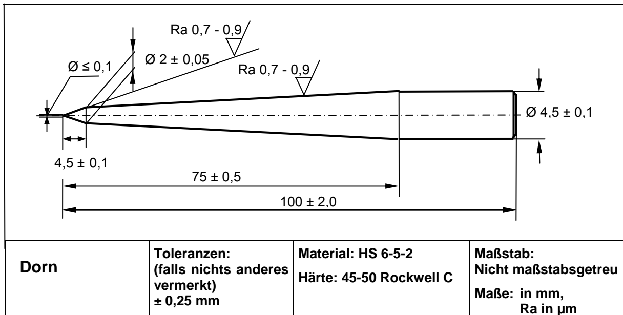
Zeichnung 2: Dorn
