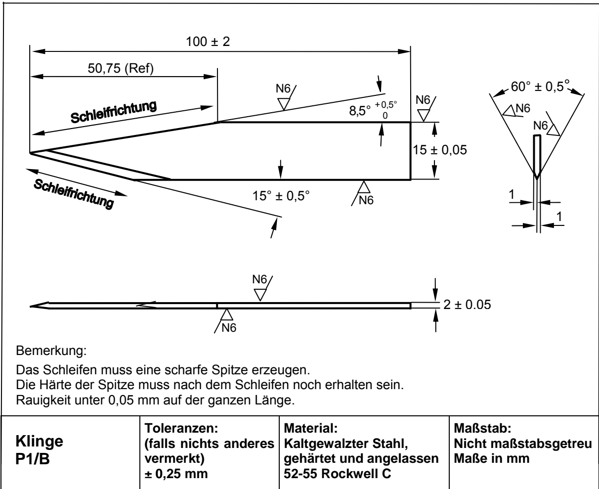
Zeichnung 1: Klinge
