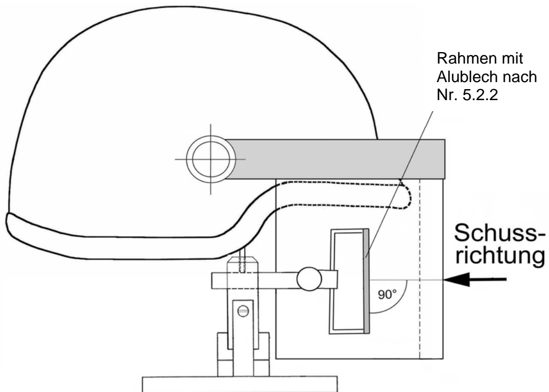
Seitenansicht schematisch
