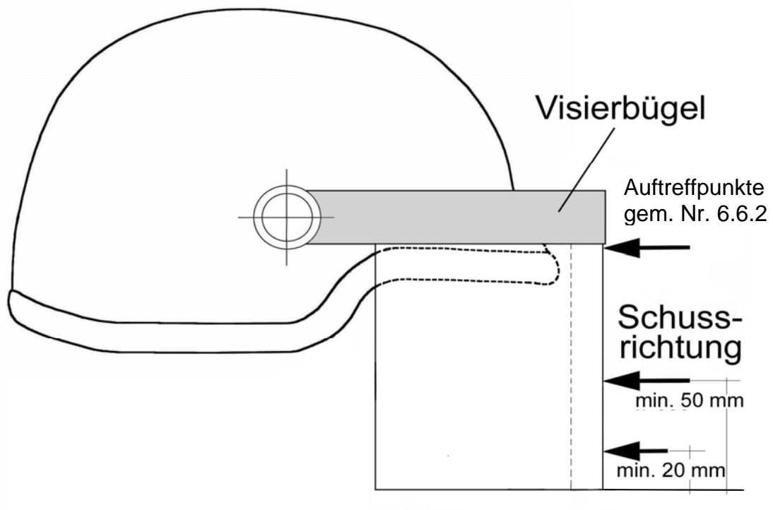
Seitenansicht
