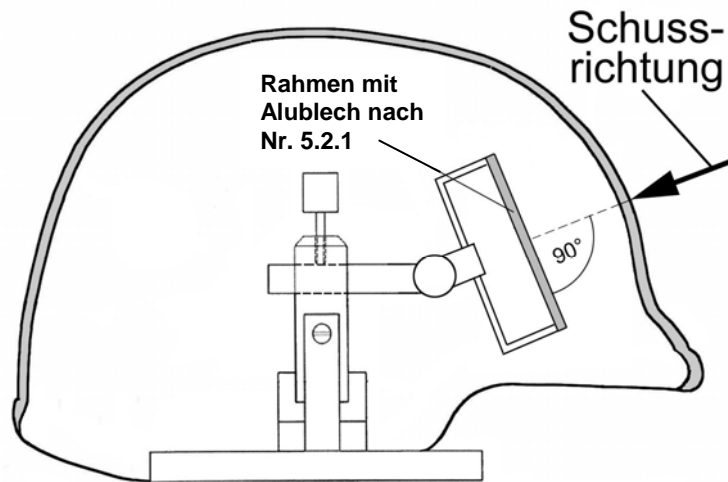
Seitenansicht
