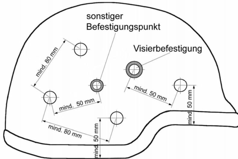
Seitenansicht
