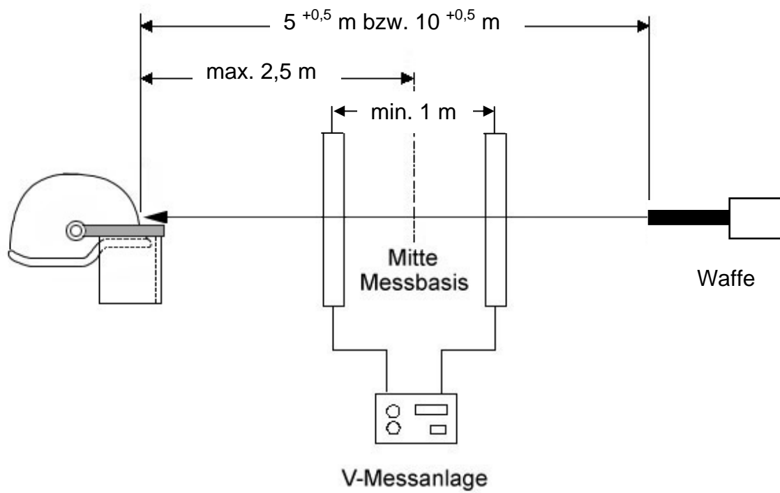
Messaufbau
